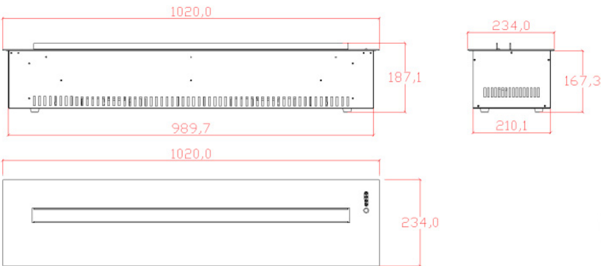
Размеры Design 1000RF 3D PS/LOG
