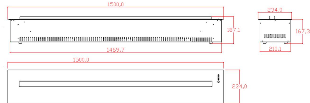
Размеры Design 1500RF 3D PS/LOG
